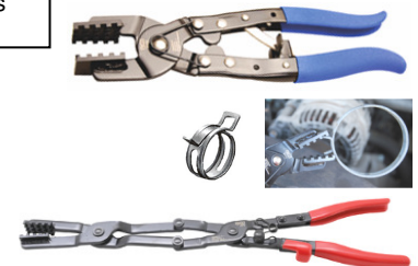
Slangklemtang - Pince pour colliers auto-serrants
