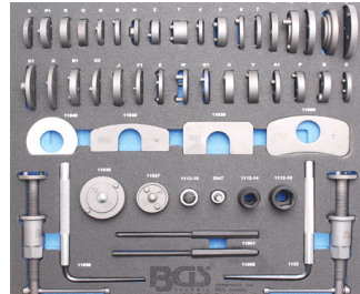
BGS1102 50 ST. / PCS. Terugstelset remzadelzuigers links-rechts 50-dlg. Set d'outils repousse piston de freins gauche-droite 50pcs 184 €
