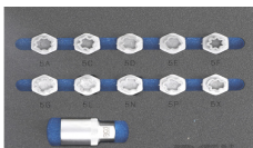
BGS9338 Doppen voor veiligheidsbouten Mercedes Douilles pour boulons de sécurité # 5A-C-D-E-F-G-L-N- P-X Class A-B-C-GLK-CLC- CLS-CLK-E-SL-SLK-M-R
